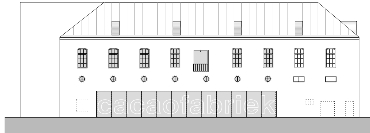
oostgevel
