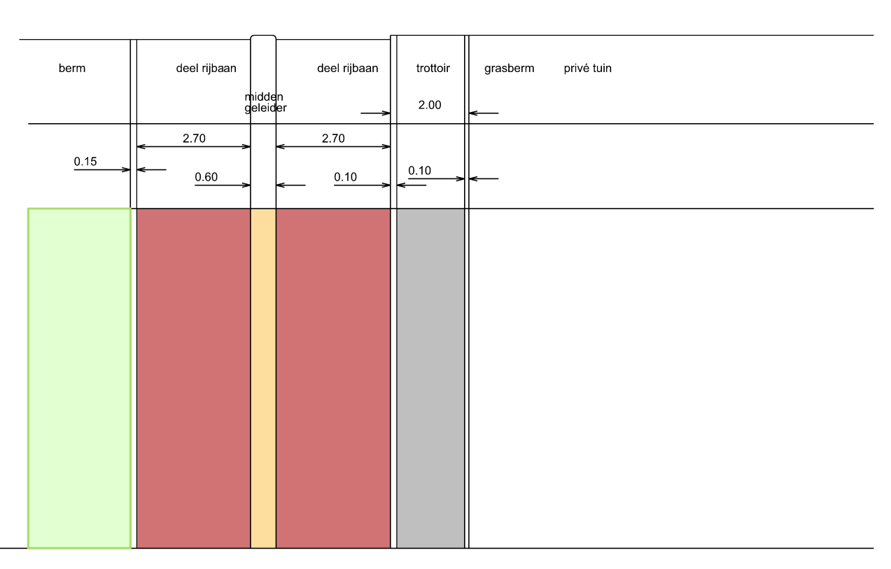
standaard profiel
